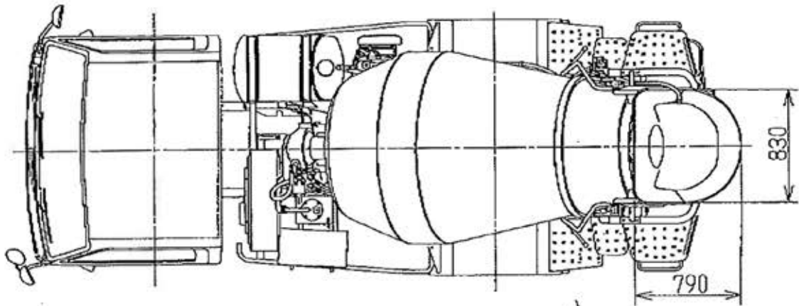
ミキサアジテータトラック外觀図 日野 2PG-XZU600H-TKFQX7 KYB MR1221(ドラム型式 M12A型 JAB1A-09001)
