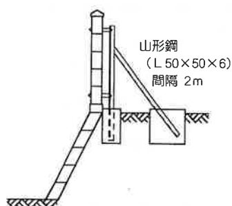
② 鋼柱(山形鋼)式
