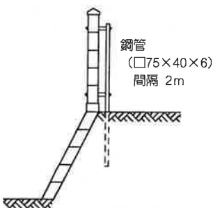
① 鋼柱(鋼管)式
